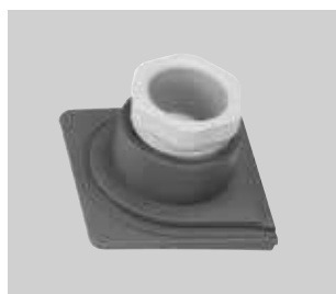
Verschraubbare Rohreinführungen M20 x 1,5
