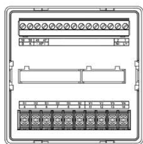
Расположение выводов
