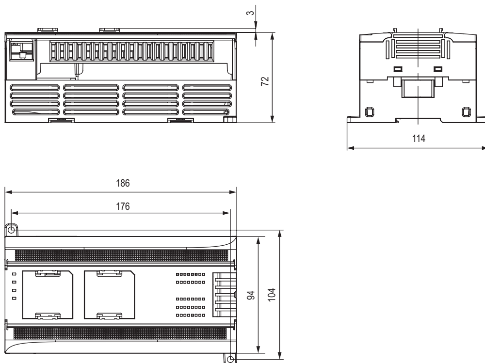
Габаритный чертеж C1000-30/C1000-40**
