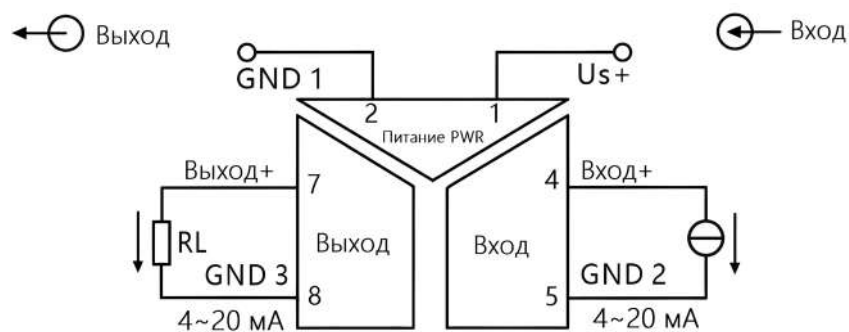
Схема подключения DSI-S-A1111
