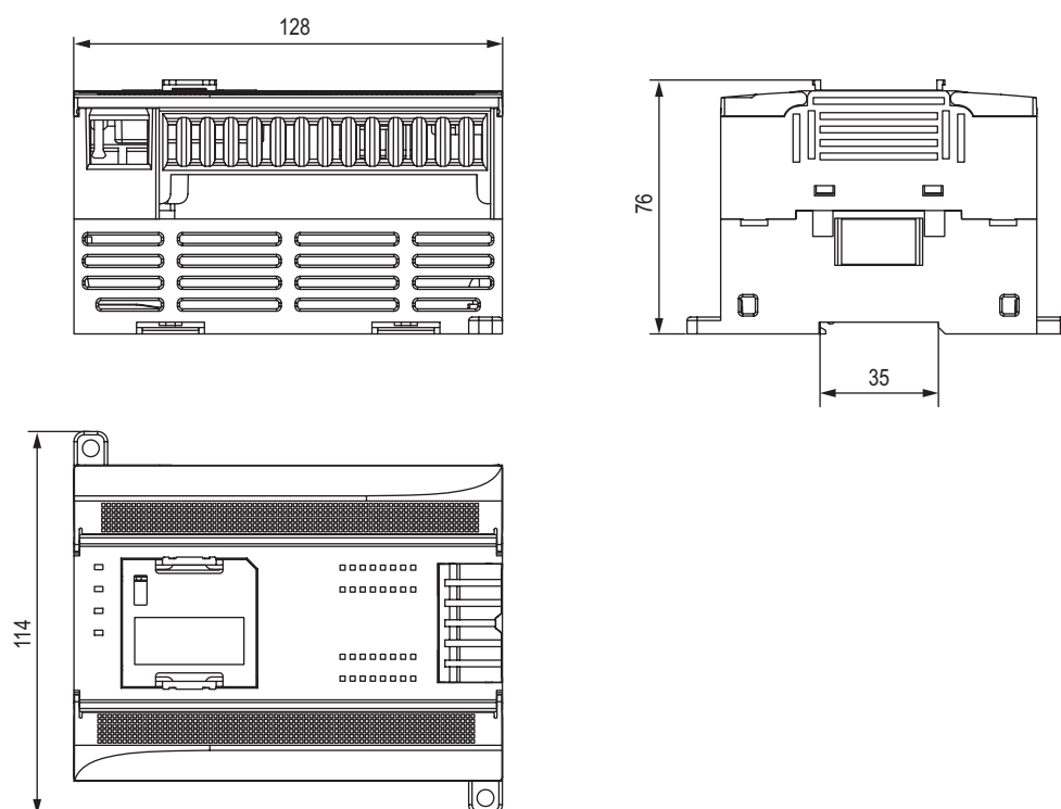
Габаритный чертеж C1000-24**
