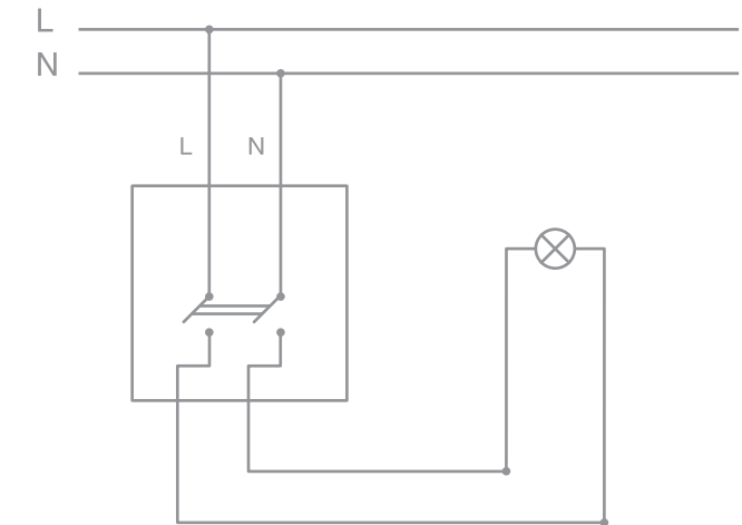
Одноклавишный двухполюсный механизм
