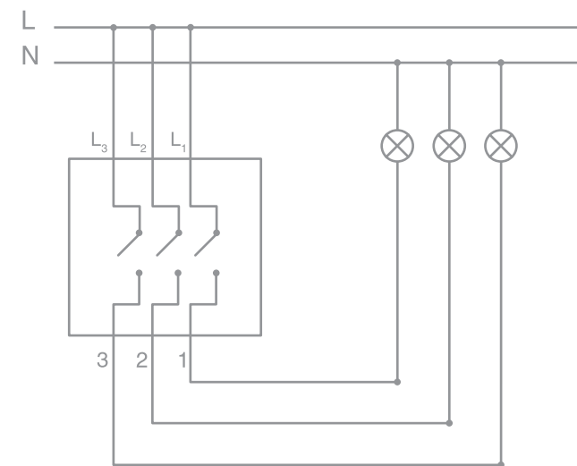
Трехклавишный выключатель
