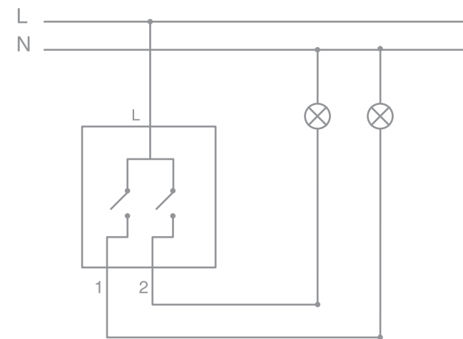
Двухклавишный выключатель
