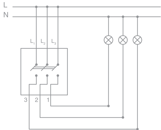
Одноклавишный трехполюсный выключатель
