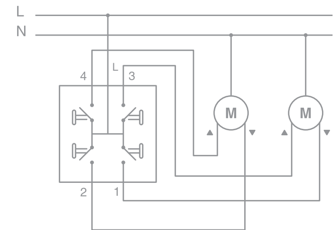
Двухклавишный механизм жалюзи
