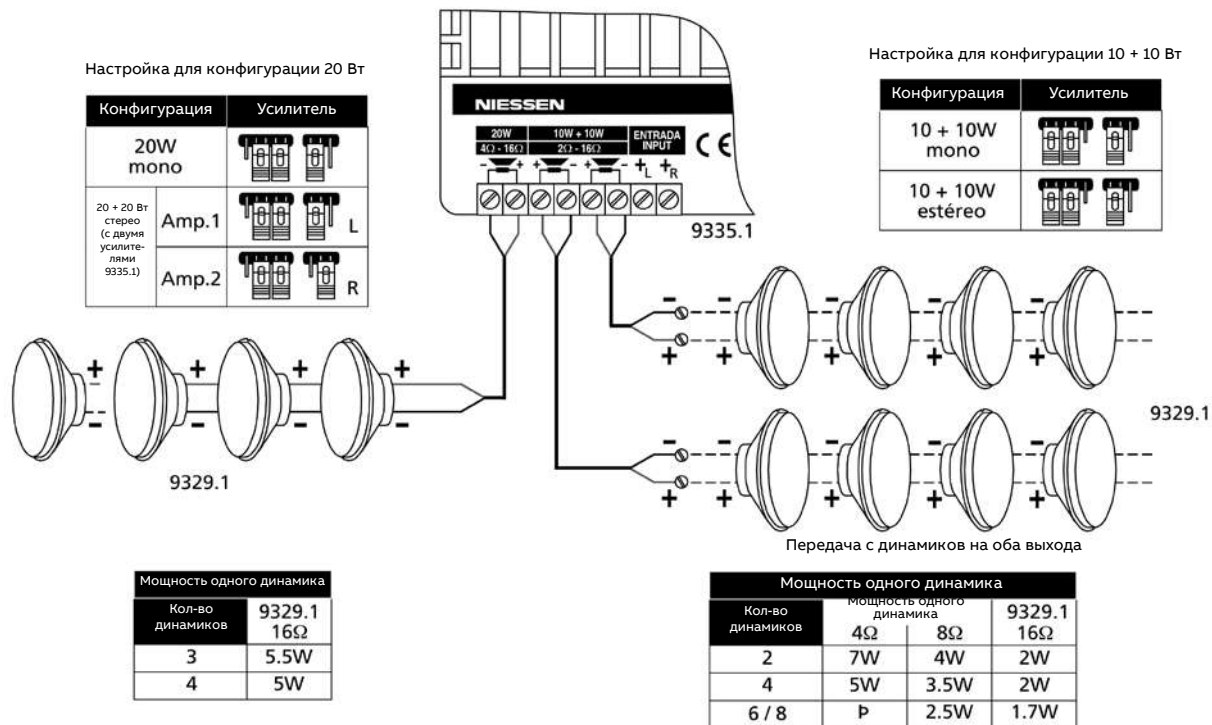
Схема подключения динамиков 9329.1 к звукоусилителю 9335.1
