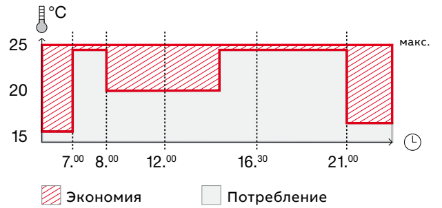
Экономия электроэнергии за счёт суточного регулирования.
